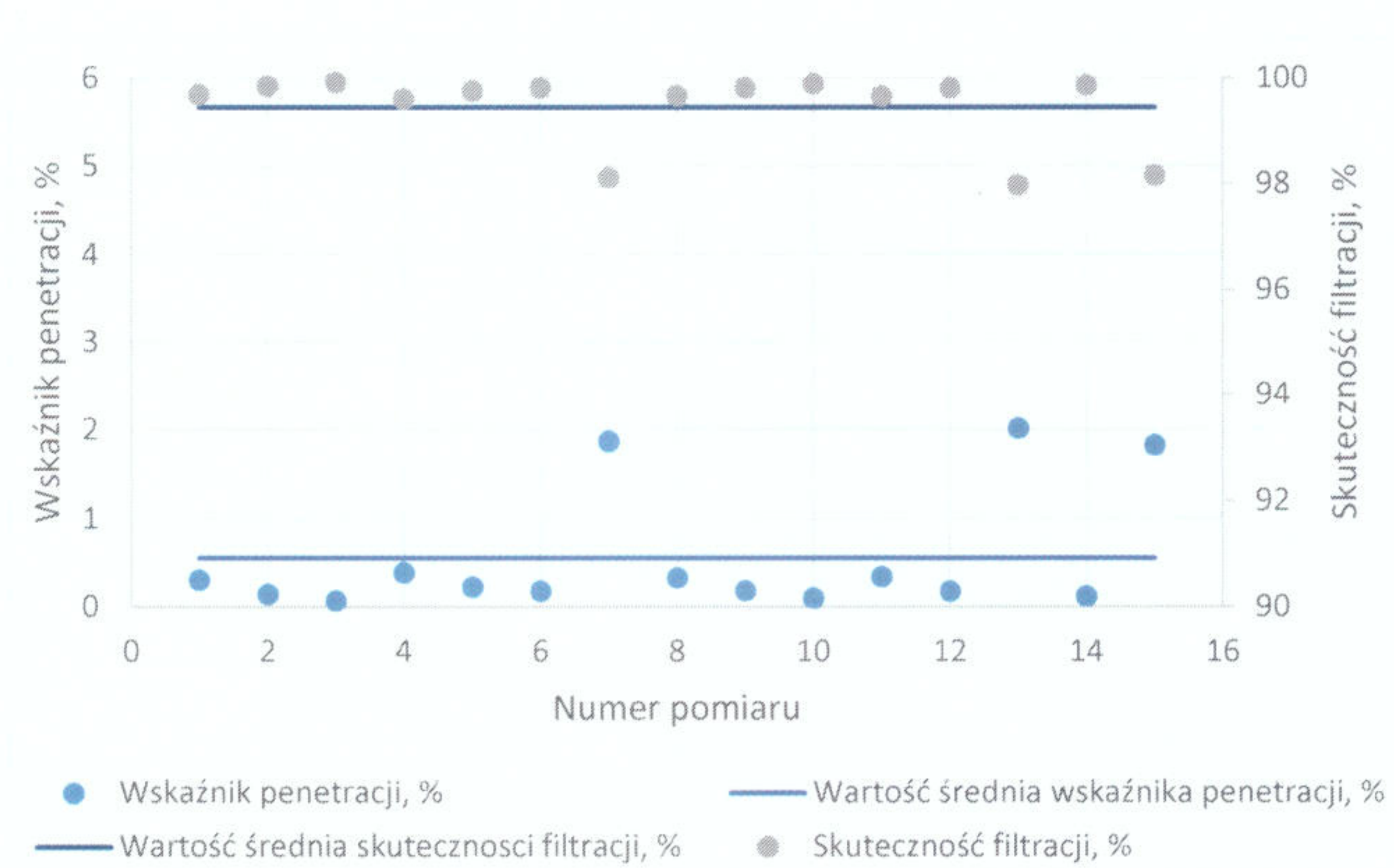
Rysunek 1 Wyniki pomiarów wskaźnika penetracji i skuteczności filtracji aerozolu chlorku sodu (frakcja pyłu PM4)
