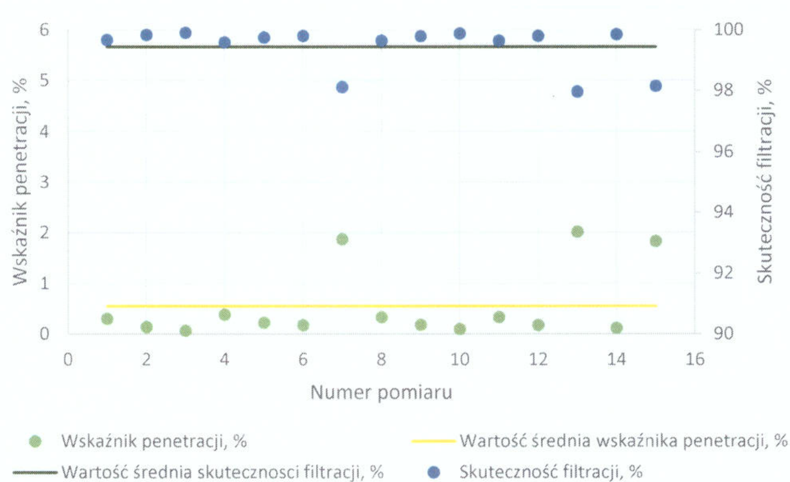
Rysunek 1 Wyniki pomiarów wskaźnika penetracji i skuteczności filtracji aerozolu chlorku sodu (frakcja pyłu PM10)
